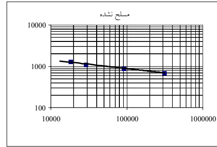
شکل ۶. منحنی خستگی برای نمونه‌های غیر مسلح
