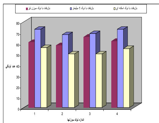
نمودار ۱. مقایسه عداد آونگی با نوک‌های مختلف
