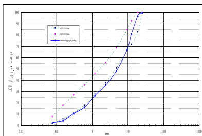
شکل ۱. مقایسه دانه بندی ترکیبی سنگدانه ها با محدوده ACI 325.10 [۱]
