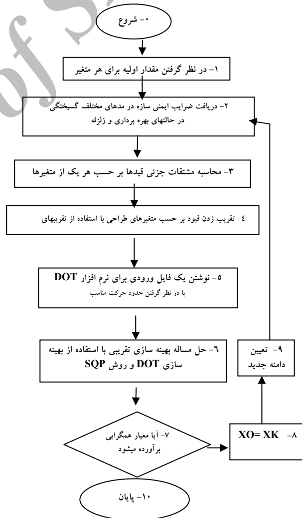
شکل ۴. الگوریتم روش بهینه سازی تقریبی
