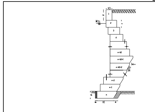
شکل ۳. متغیرهای طراحی و شکل کلی مقطع گویشتی مورد مطالعه
