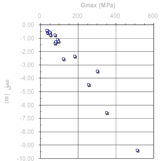
شکل ۵. نمودار تغییرات سختی بر حسب عمق در نقطه ۱
