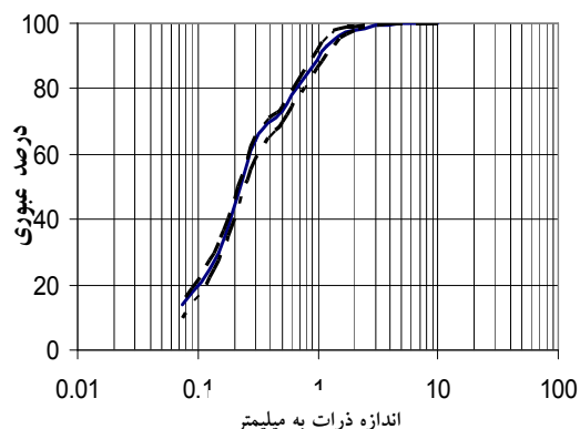
شکل ۱. پوش دانه‌بندی مصالح بستر در محل آزمایش
