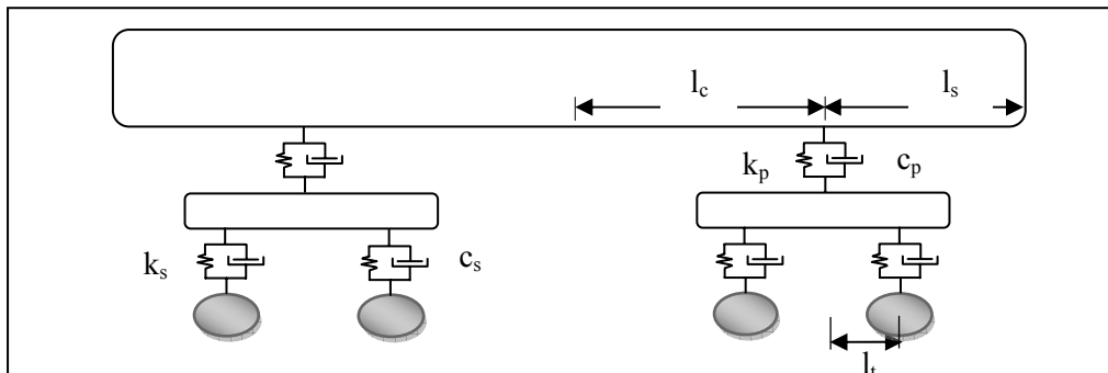
شکل ۱. مدل دوبعدی از واگن قطار
