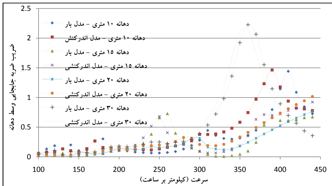
شکل ۸. ضربه جانبی وسط دهانه
