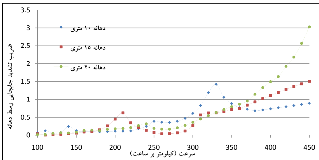
شکل ۱۰. ضربه ضربه جابجایی وسط دهانه
