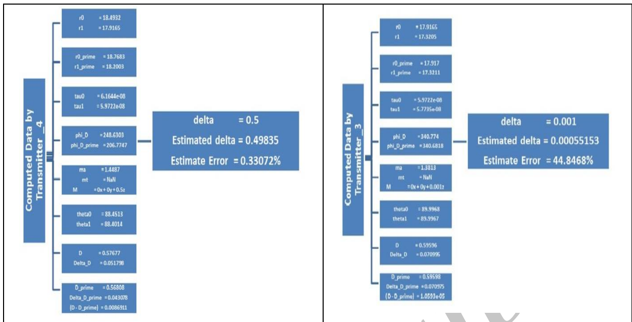
شکل 9. اطلاعات محاسباتی و شبیه سازی مربوط به فرستنده سه
