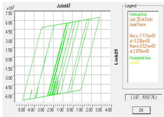
شکل 24. نمودار هیستریک میراگر پیرامونی
