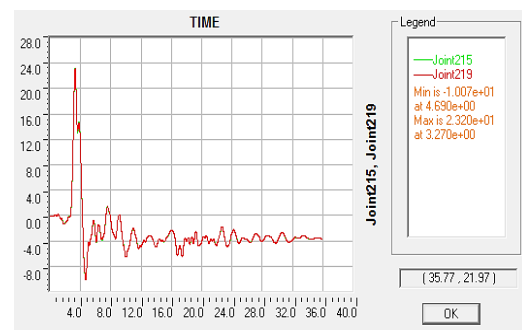
شکل 22. نمایش عدم پیش در سازه هشت طبقه
