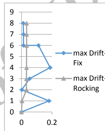
شکل 32. نمایش دررفت در سازه 8 طبقه در دو حالت گهواره‌ای و حالت گیردار
