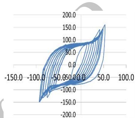
شکل 7. نمودار هیستریک استخراجی مدل آزمایشگاهی
