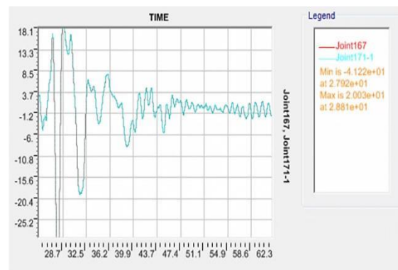
شکل 17. نمایش عدم پیچش در سازه هشت طبقه
