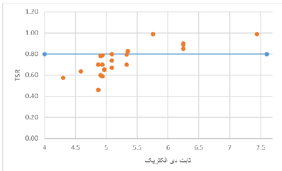
شکل ۹. نمودار رابطه TSR و ثابت دی الکتریک
