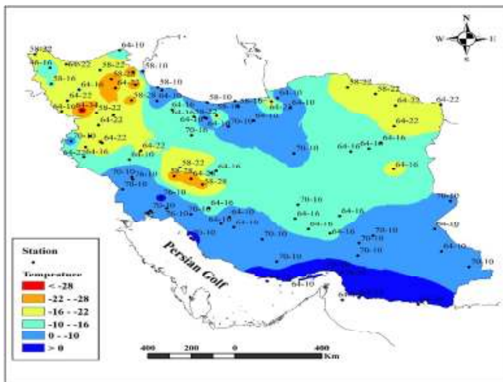
شکل ۲. پهنه‌بندی حرارتی (دمای پائین) روسازی به منظور تعیین PG بر حسب درجه سانتی گراد
