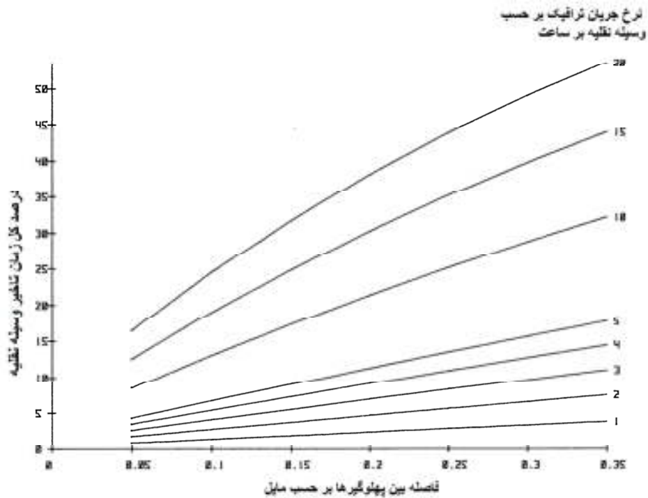
شکل ۶. نمودار درصد کل زمان تاخیر-فاصله بین پهلوگیرها در راه‌های یک خطه دو طرفه (Anderson, 1980)
