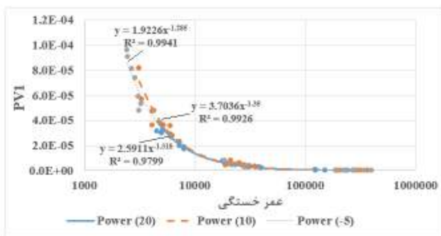
شکل ۱۲. ارتباط بین عمر خستگی و PVI برای نمونه‌های مسلح شده در دماهای مختلف در فرکانس ۱۰ هرتز
