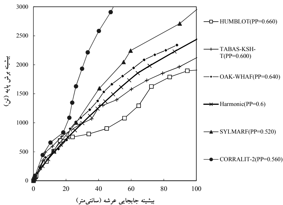
شکل ۲۱. نتایج تحلیل‌های دینامیکی فزاینده با شتاب‌نگاشت زلزله و هارمونیک (دوره تناوب غالب شتاب‌نگاشت = 0.76 - 0.52 )
