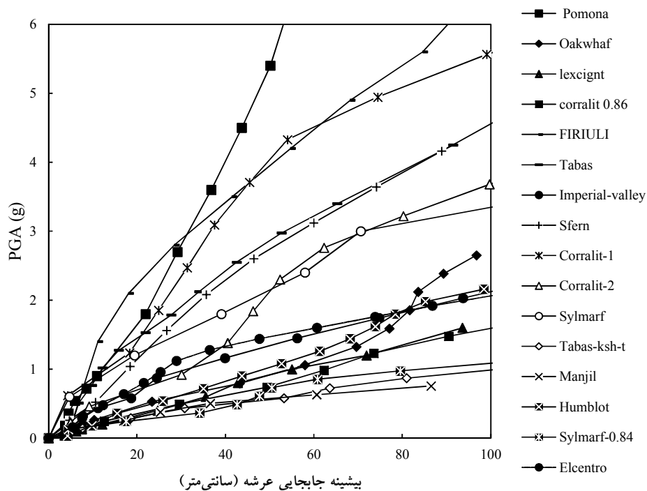
شکل ۱۳. نتایج تحلیل دینامیکی فزاینده مدل دوم بر حسب معیار شدت PGA
