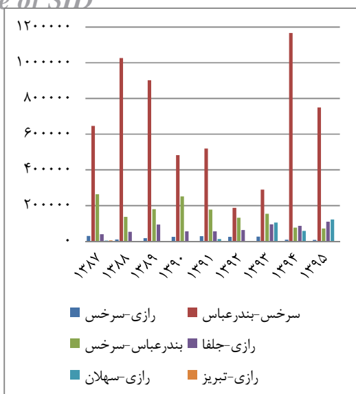
نمودار ۱. کالاهای ترانزیتی حمل شده محورهای مختلف در بخش حمل و نقل ریلی کشور طی سال‌های ۹۵-۱۳۸۷
