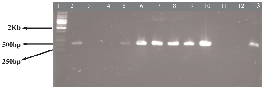
شکل ۱: محصول PCR، آغازگر cagA-Ir ، الکتروفورز شده در آگارز یک درصد. چاهک شماره ۱ مارکروزن ملکولی ۱Kb، چاهک شماره ۲ شاهد مثبت، چاهک شماره ۳ شاهد منفی، چاهک‌های شماره ۵، ۶، ۷، ۸، ۹، ۱۰، ۱۳ نمونه‌های cagA مثبت و چاهک‌های شماره ۴، ۱۱ و ۱۳ نمونه‌های منفی cagA .
