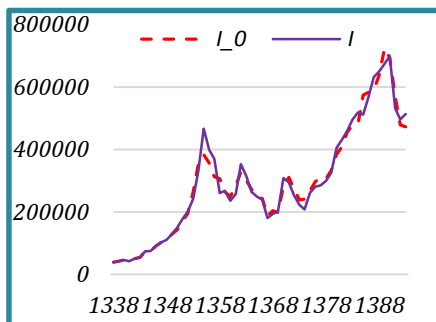
نمودار ۳. شبیه‌سازی سرمایه‌گذاری کل
