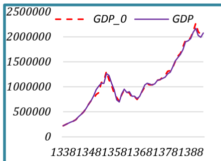
نمودار ۴. شبیه‌سازی تولید ناخالص داخلی
