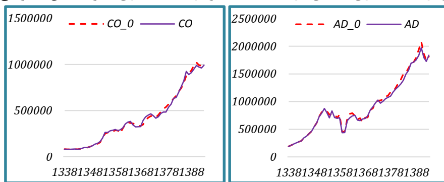
نمودار ۱. شبیه سازی تقاضای کل نمودار ۲. شبیه سازی مصرف بخش خصوصی
