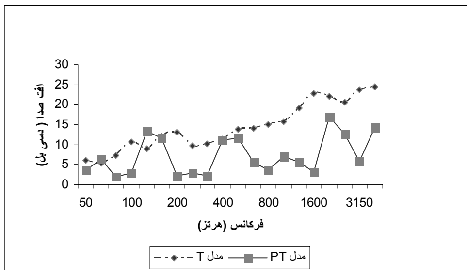
شکل ۴- مقایسه افت صدا در دو مانع مدل T و PT در محل گیرنده (0, -50)
