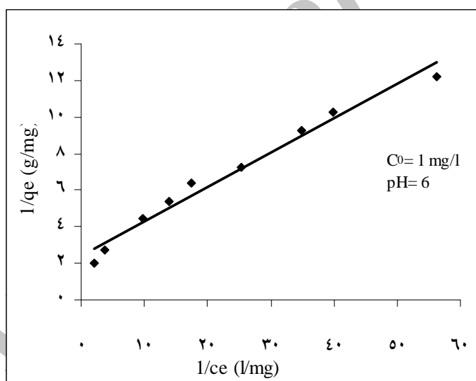
نمودار ۶- رسم خطی مدل ایزوترم Langmuir جذب سرب توسط جاذب پوسته شلتوک
