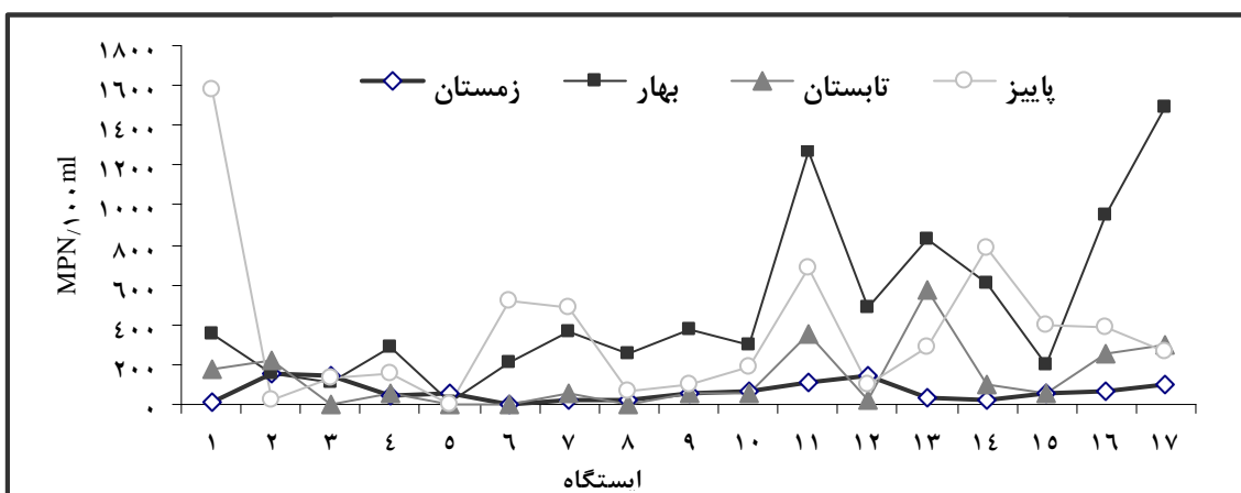
نمودار ۳- تغییرات میانگین E.coli در ایستگاه های مورد مطالعه در فصول مختلف سال
