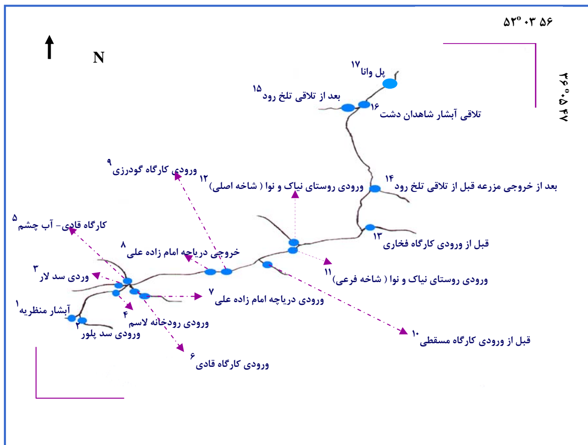
شکل ۲- موقعیت ایستگاه‌های مورد مطالعه در رودخانه هراز
