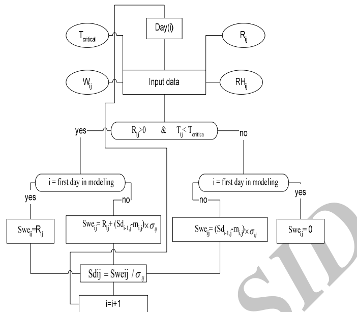
شکل ۳- الگوریتم محاسبه ارتفاع آب معادل برف در مدل SWEG
