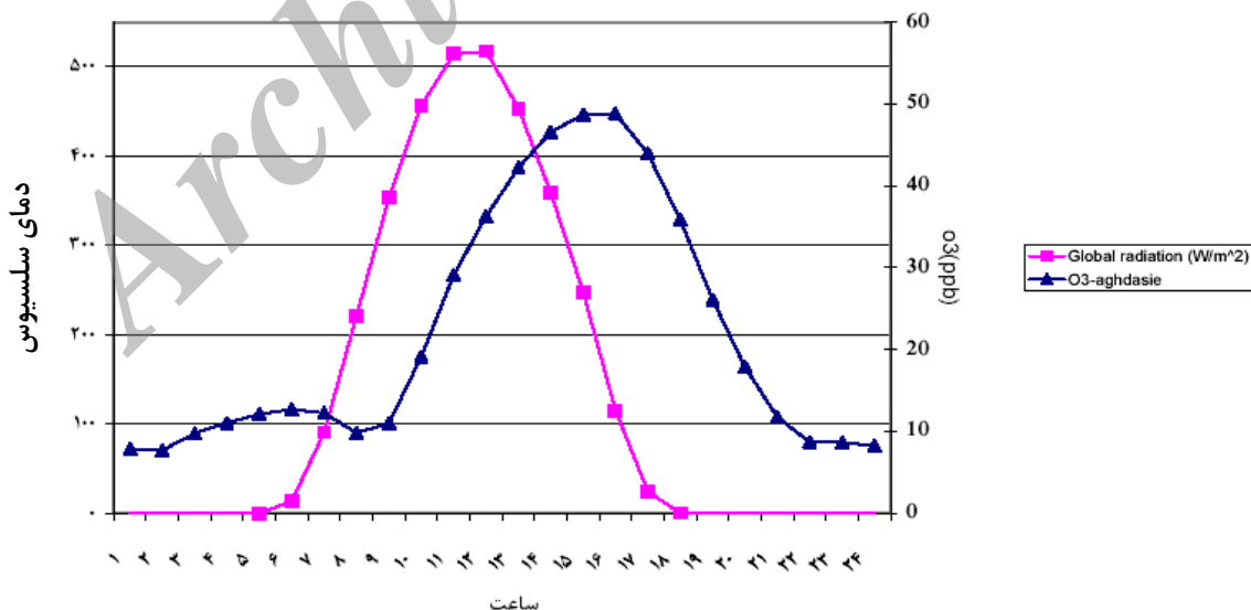
نمودار ۲- تغییرات میانگین ساعتی غلظت ازن با تغییرات میانگین ساعتی
