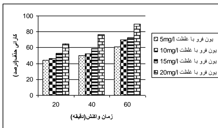
نمودار ۴- کارایی حذف دترجنت ستیل تری متیل آمونیوم بروماید در pH=4 ، غلظت ۵۰ میلی لیتر پروماید (C-TAB) با استفاده از فرآیند فنتون در pH=4 و بررسی تاثیر زمان ماند، مقدار یون فرو و مقدار پراکسید هیدروژن مورد بررسی قرار گرفته است. نتایج حاصل از تحقیقات انجام شده نشان داده است که میزان حذف دترجنت در pH پایین، افزایش قابل ملاحظه ای می یابد (۱۱ و ۱۰). تحقیقات گذشته نیز ثابت کرده اند که کارایی حذف دترجنت ها در شرایط اسیدی ( pH=3-5 ) بسیار سریع اتفاق می افتد (۱۱ و ۱۳). در pH پایین تر از ۲/۵ تشکیل Fe(OH)^{+2} که با هیدروژن پراکسید به آرامی واکنش می دهد باعث کاهش مقدار رادیکال های OH^0 شده و در نتیجه بازدهی فرآیند کاهش می یابد. در pH های قلیایی نیز Fe^{+2} به Fe^{+3} تبدیل شده و به صورت Fe(OH)_3 رسوب می کند و از چرخه کاتالیستی حذف می شود. این مساله خود باعث تجزیه هیدروژن پراکسید و کاهش بازدهی فرآیند می شود. هم چنین تحقیقات نشان داده اند که پتانسیل اکسایشی رادیکال های هیدروکسیل با افزایش pH کاهش می یابد (۱۱ و ۱۳). از طرفی با افزایش زمان ماند، افزایش غلظت یون فرو و پراکسید هیدروژن کارایی حذف دترجنت افزایش می یابد (۹ و ۱۰). با توجه به نتایج به دست آمده از این تحقیق کاربرد فرآیند فنتون در جهت حذف دترجنت ها در pH اسیدی ( pH=4 ) پیشنهاد می گردد. دلیل عمده آن خوردگی و انحلال بیشتر یونهای Fe^{+2} در محیط اسیدی و افزایش تولید رادیکال OH^0 می باشد. کارایی حذف دترجنت ها با افزایش غلظت یون فرو و افزایش غلظت پراکسید هیدروژن افزایش می یابد، به
