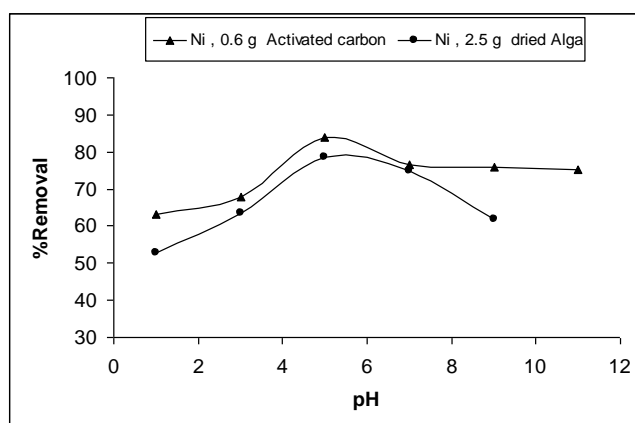
شکل ۱- اثر جذب در pH بین ۹-۱ محلول نمک \text{NiCl}_2 \cdot 6\text{H}_2\text{O} (97%)
