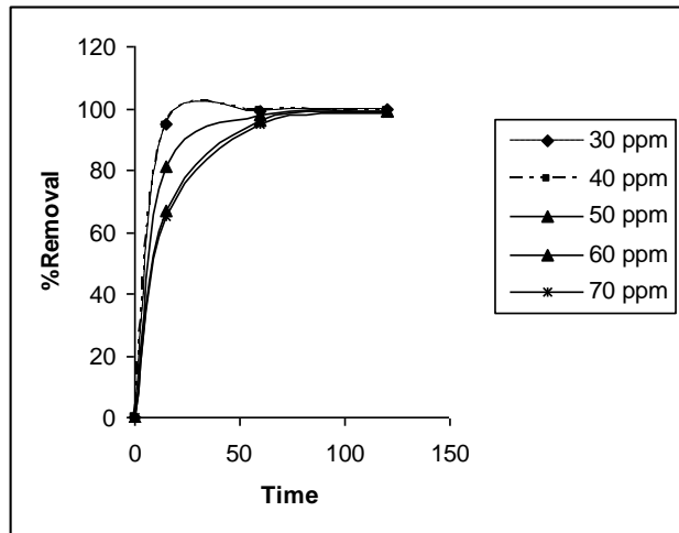
شکل ۲- اثر زمان نسبت به غلظت های متفاوت محلول نمک NiCl_2 \cdot 6H_2O (۹۷٪) در pH = 5 و 0.6 گرم جاذب
