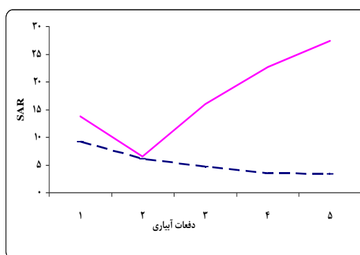
شکل ۵- روند تغییرات SAR در عصاره اشباع خاک بر اساس دفعات آبیاری با آب چاه و پساب خروجی از تصفیه‌خانه پرکنند آباد، خط ممتد آبیاری با پساب و خط منقطع آبیاری با آب چاه می‌باشد
