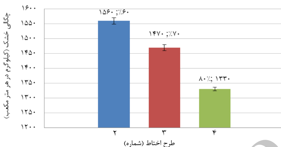
شکل ۱۰- چگالی خشک متوسط بتن شامل پسماند نوع ۱۰
