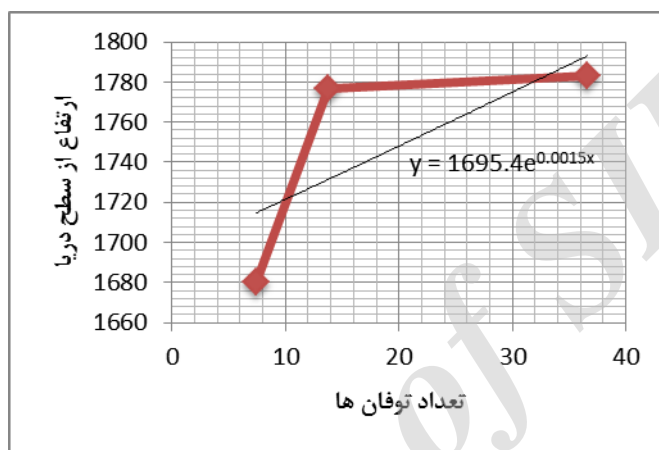
شکل 8- تغییرات وقوع توفان های گردو غبار با ارتفاع از سطح دریا
