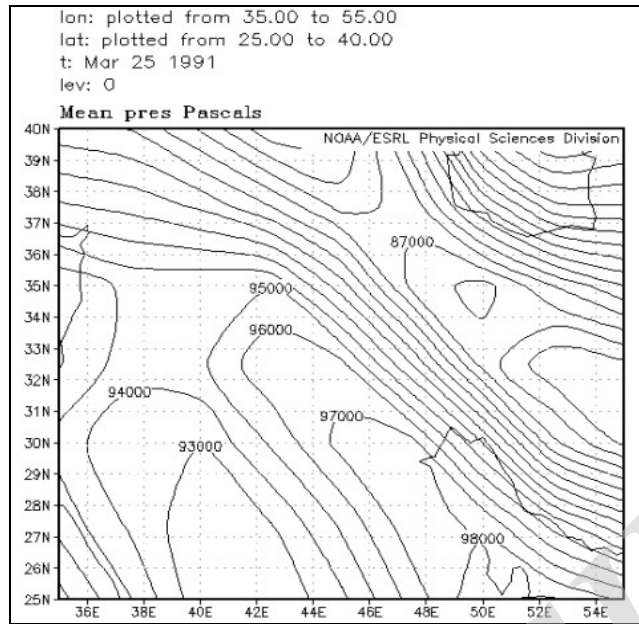
شکل 14- الگوی فشار سطح زمین - 25 مارس 1991 میلادی
