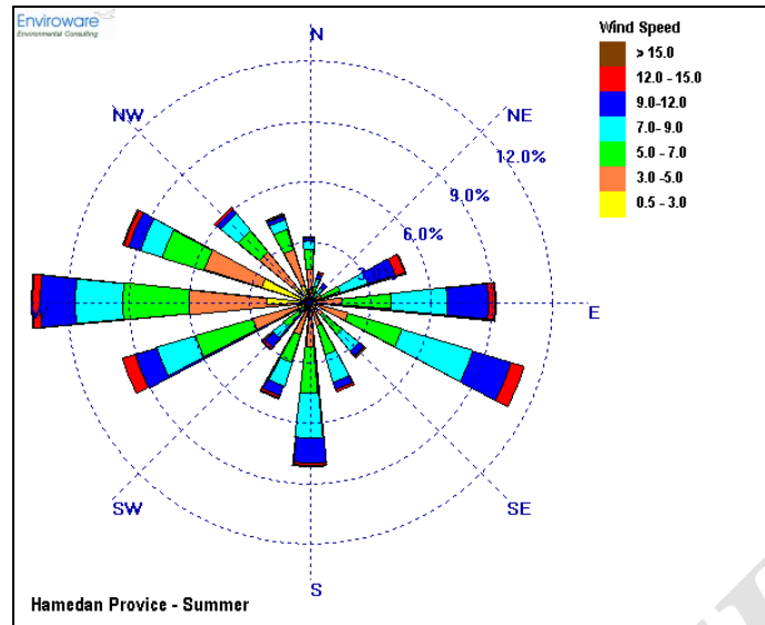
شکل 18- گلباد فصل تابستان منطقه مورد مطالعه
