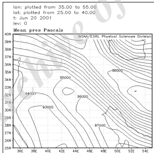
شکل 15- الگوی فشار سطح زمین - روز 20 ژوئن 2001 میلادی
