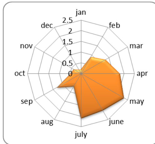
شکل 3- نمودار تغییرات میانگین ماهیانه توفان های گردو غبار ایستگاه ملایر در دوره 1992 تا 2010 میلادی
