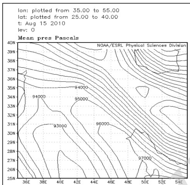
شکل 16- الگوی فشار سطح زمین - روز 15 اوت 2010 میلادی
