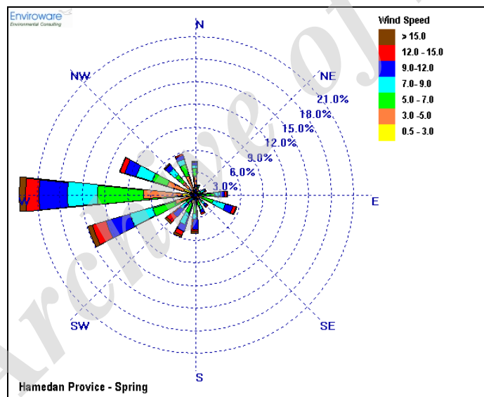
شکل 17- گلباد فصل بهار برای منطقه مورد مطالعه
