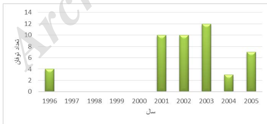
شکل 4- نمودار تغییرات توفان های گردو غبار ایستگاه نهاوند در دوره 1996 تا 2005 میلادی
