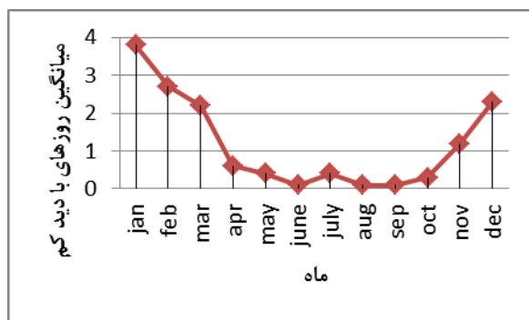
شکل 9- میانگین ماهیانه روزهای با دید کم تر از 2 کیلومتر در ایستگاه ملایر (دوره آماری 1992 تا 2010 میلادی)
