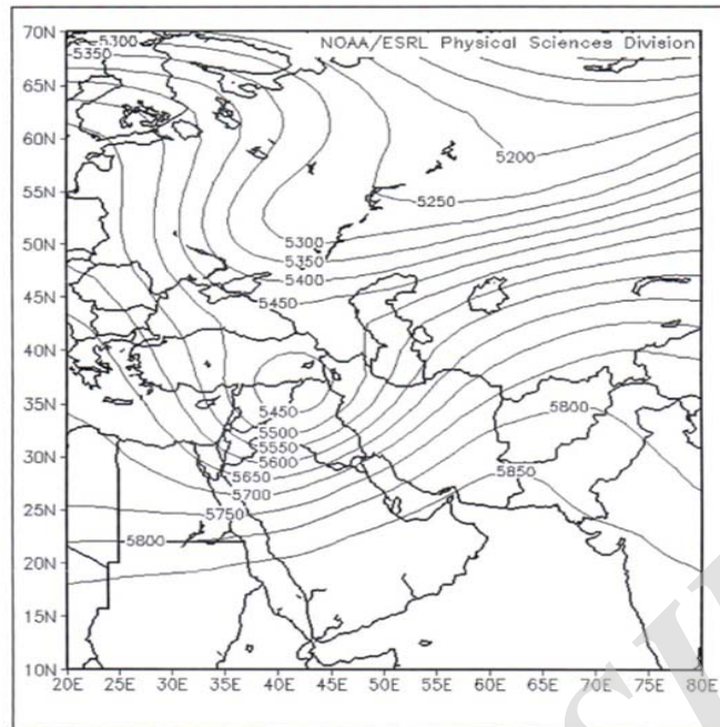
شکل 13- الگوی تراز 500 هکتوپاسکال - 26 مارس 2003 میلادی
