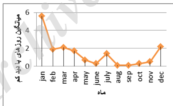
شکل 11- میانگین ماهیانه روزهای با دید کم تر از 2 کیلومتر در ایستگاه تويسرکان (دوره آماری 2004 تا 2010 میلادی)
