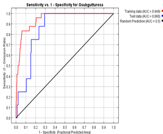
شکل 2- منحنی ROC
