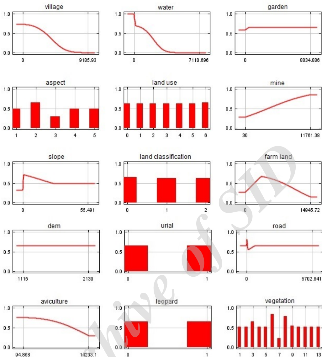
شکل 3- منحنی های پاسخ
