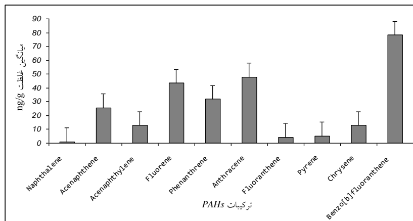
شکل ۳- غلظت میانگین (±انحراف معیار) فردی ترکیبات PAH در رسوبات سیسنگان (نانوگرم بر گرم وزن خشک)
