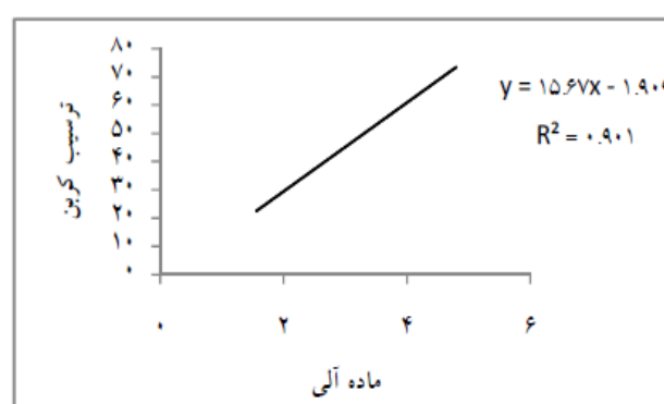
شکل ۶- رابطه رگرسیونی بین ترسیب کربن سرو نقره‌ای و ماده آلی Cupressus arizonica Green. and organic mater
