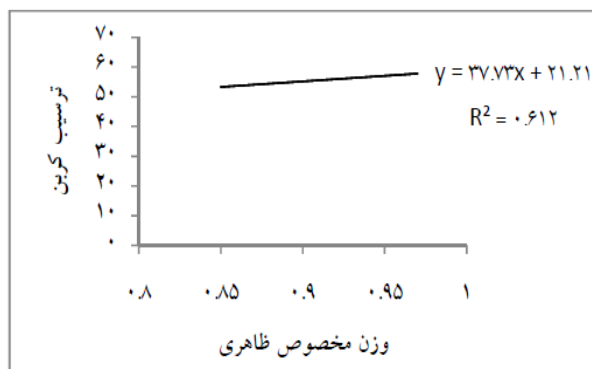
شکل ۵- رابطه رگرسیونی بین ترسیب کربن کاج تهران و وزن مخصوص ظاهری Pinus eldarica Medw. and Bulk density
