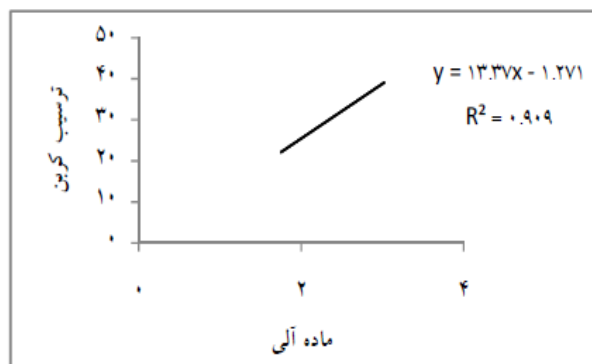
شکل ۹- رابطه رگرسیونی بین ترسیب کربن بلوط ایرانی و ماده آلی Quercus brantii Lindl. and organic mater
