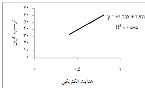
شکل ۴- رابطه رگرسیونی بین ترسیب کربن کاج تهران و هدایت الکتریکی Pinus eldarica Medw. and The electrical
