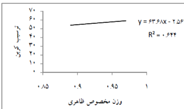
شکل ۸- رابطه رگرسیونی بین ترسیب کربن سرو نقره‌ای و وزن مخصوص ظاهری Cupressus arizonica Green. and Bulk density
