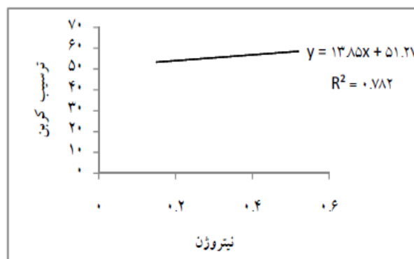
شکل ۷- رابطه رگرسیونی بین ترسیب کربن سرو نقره‌ای و نیتروژن Cupressus arizonica Green. and nitrogen
