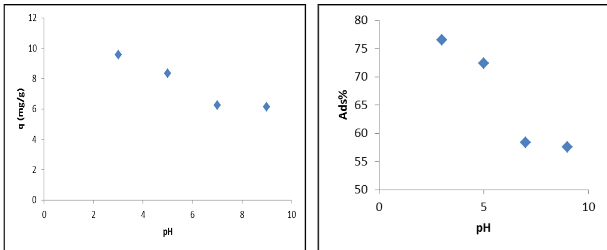
شکل ۳- اثر پارامتر pH بر درصد جذب و ظرفیت جذب فسفات توسط اکسید گرافن
