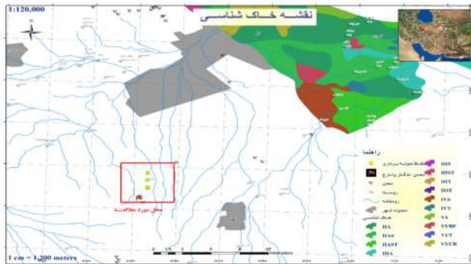
شکل ۱ - محل های نمونه برداری از خاک های اطراف معدن منگنز و نارچ قم در سه نقطه به فواصل یک کیلومتر (۱۰) Figure 1- Sampling places from the Surrounding Soils of Venarch Manganese Mine in Qom in tree points.
