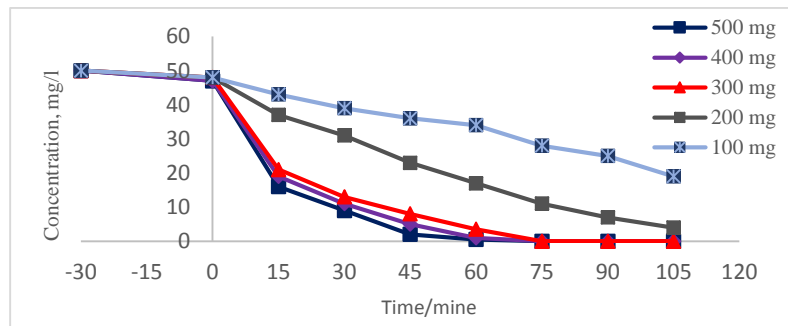
نمودار ۷- اثر غلظت فوتوکاتالیست تحت نور UV Figure 7. The effect of Photocatalysts concentration under UV light
