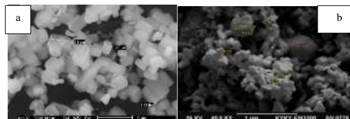
شکل ۴- تصاویر SEM (الف) زئولیت Fe-ZSM-5، (ب) فوتوکاتالیست Fe-ZSM-5@TiO 2 _Ag
