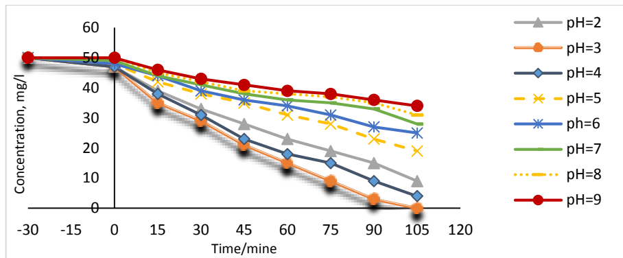
نمودار ۸- اثر pH در حذف رنگ تحت نور UV
