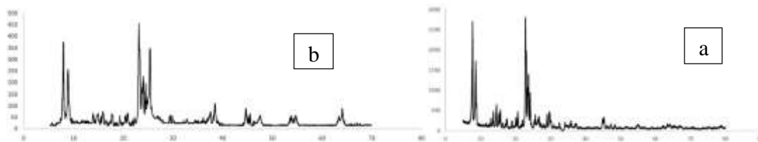
شکل ۳ - الگوی XRD (الف) زئولیت Fe-ZSM-5، (ب) فوتوکاتالیست Fe-ZSM-5@TiO 2 _Ag
