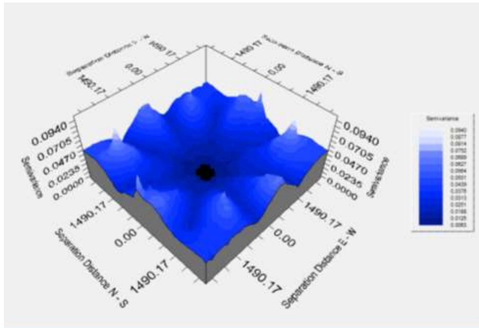
شکل ۸- نمودار سمی واریوگرام سه بعدی لگاریتم Cd
