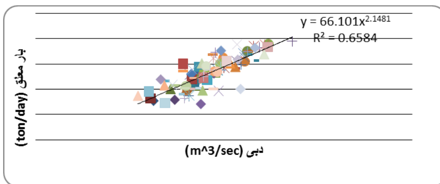
شکل ۳- ساخت مدل به کمک منحنی سنجهی رسوب در ایستگاه قرآن تالار
