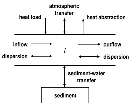
شکل ۵- موازنه دما
