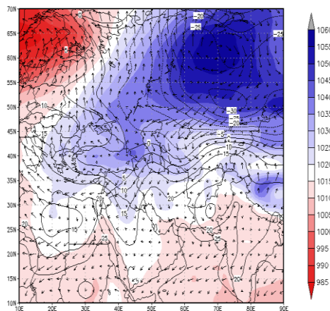
الف - روز ۲۹ آبان ماه
