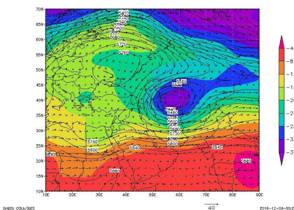
ج- روز ۳ آذرماه
