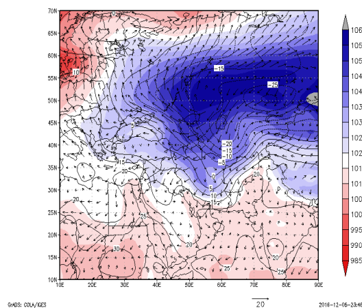
پ - روز ۱ آذرماه
