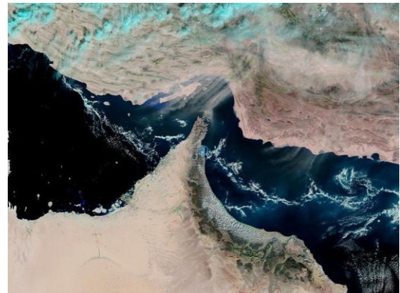
الف- تصاویر ماهواره مودیس ۱ آذرماه
