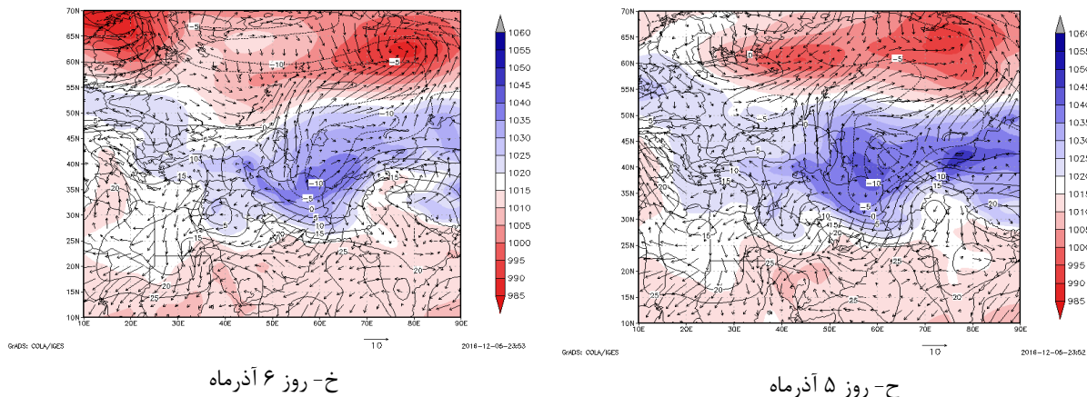
شکل ۲- نقشه ترکیبی فشار تراز دریا (میلی بار)، بردار باد (متر بر ثانیه) و دما (سلسیوس) در روزهای
