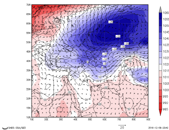
ب - روز ۳۰ آبان ماه
