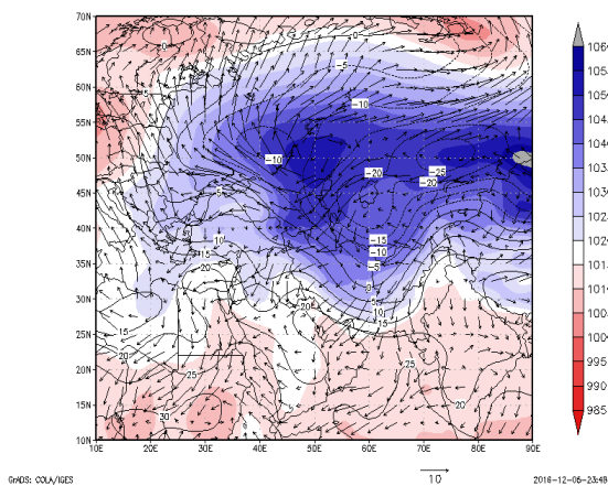
ت - روز ۲ آذرماه
