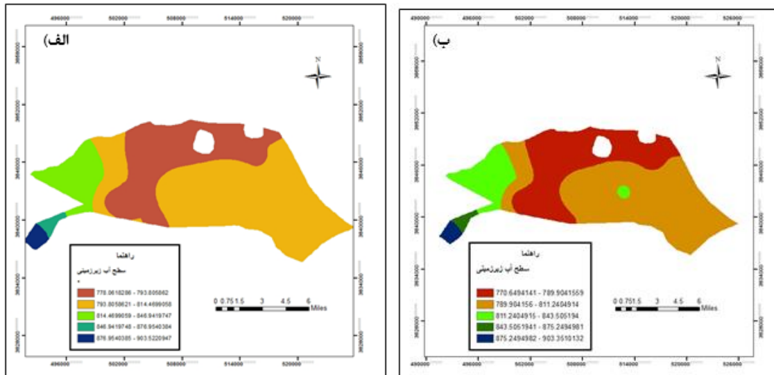
شکل ۲- پهنه بندی سطح آب زیرزمینی در حوزه آبخیز شریف آباد (الف) سال ۱۳۸۷ و (ب) سال ۱۳۹۳
