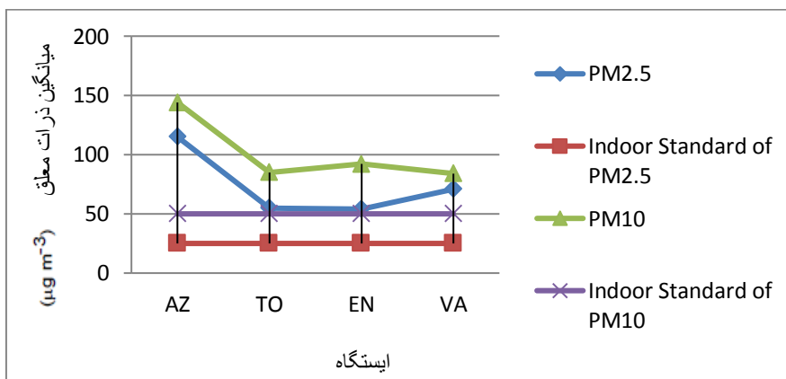
شکل ۵- میانگین غلظت های PM_{10} و PM_{2.5} در ایستگاه های زیرزمینی متروی شهر تهران در فصل بهار ۱۳۹۵
