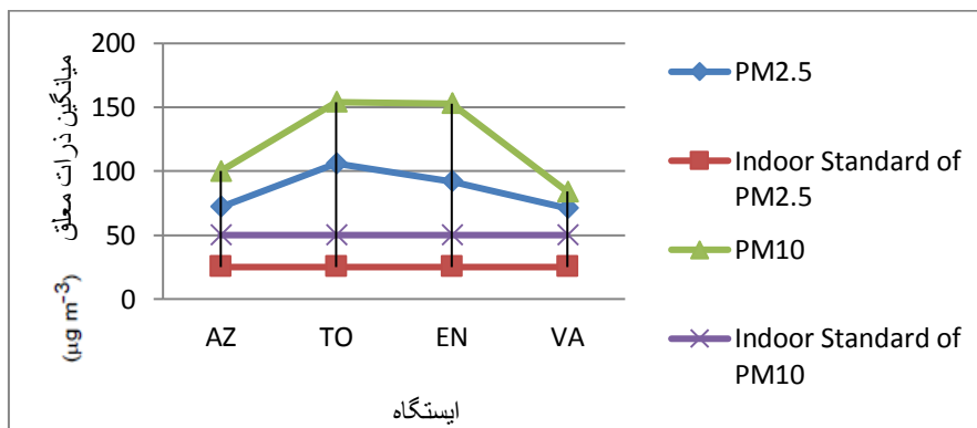
شکل ۴- میانگین غلظت های PM_{10} و PM_{2.5} در ایستگاه های زیرزمینی متروی شهر تهران در فصل زمستان ۱۳۹۵
