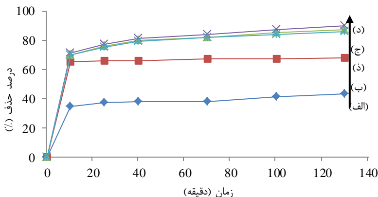
شکل ۵- فعالیت فتوکاتالیستی نانوذرات دی اکسید تیتانیوم (الف)، نانوکامپوزیت دی اکسید تیتانیوم / بنتونیت اولیه (ب) و دوپ شده با ۳ (ج)، ۵ (د)، ۱۰ درصد نقره در حضور نور مرئی.
