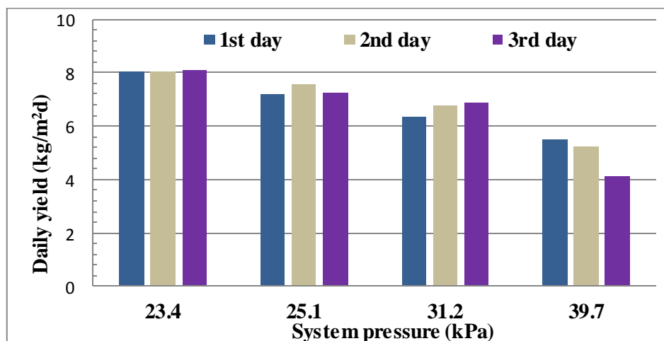
نمودار ۴- اثر فشارهای مختلف سیستم بر میزان آب تولیدی در سه روز متوالی (آزمایش دوم)
