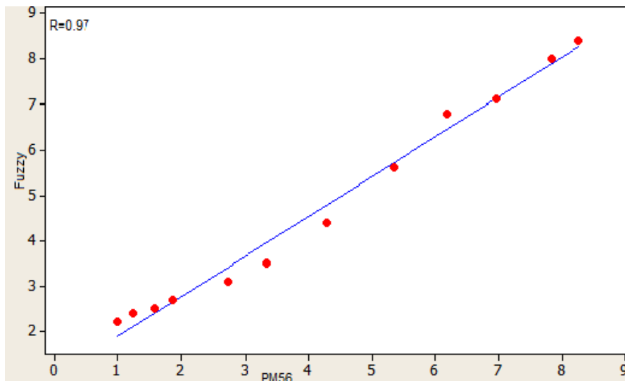
شکل ۲- مقایسه برآورد تبخیر و تعرق با مدل فازی ممدانی و مدل پنمن - مانتیث - فائو
