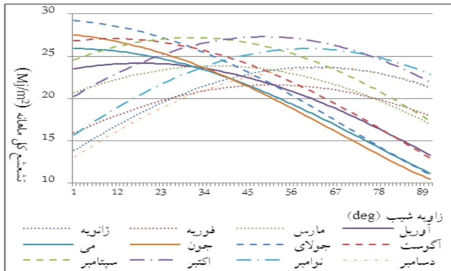
نمودار ۱- مقدار تشعشع کل روی سطوح شیب‌دار به صورت ماهانه Chart 1- The total radiation on tilted surfaces of each month
