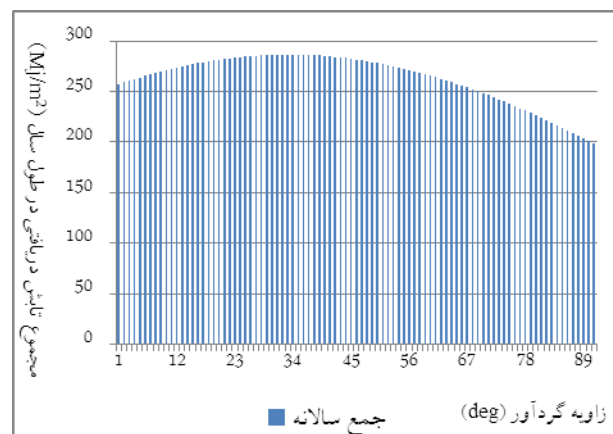
نمودار ۴- جمع سالانه تشعشع کل بر روی سطوح شیب‌دار بر حسب زاویه برای شهر کرمان
