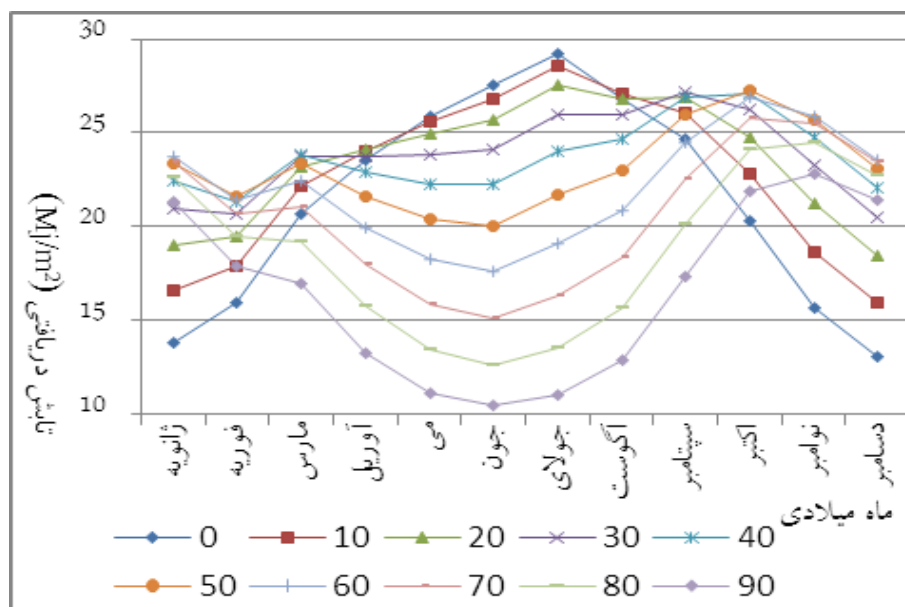
نمودار ۲- مقدار تابش دریافتی برای زوایای شیب ۰ الی ۹۰ درجه برحسب مگاژول بر متر مربع برای شهر کرمان در ماه‌های سال Chart 2- Received radiation ( Mj/m^2 ) on tilted angles of 0 to 90 of each month in Kerman
