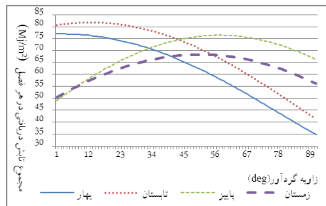
نمودار ۳- تشعشع کل روی سطح شیب‌دار بر حسب زاویه به صورت فصلی برای شهر کرمان
