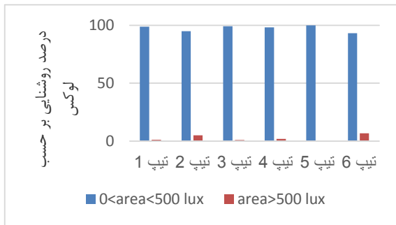
شکل ۱۹- نتایج آنالیز شبیه سازی میزان روشنایی در روز اول تابستان ساعت ۱۲ ظهر (نگارندگان)
