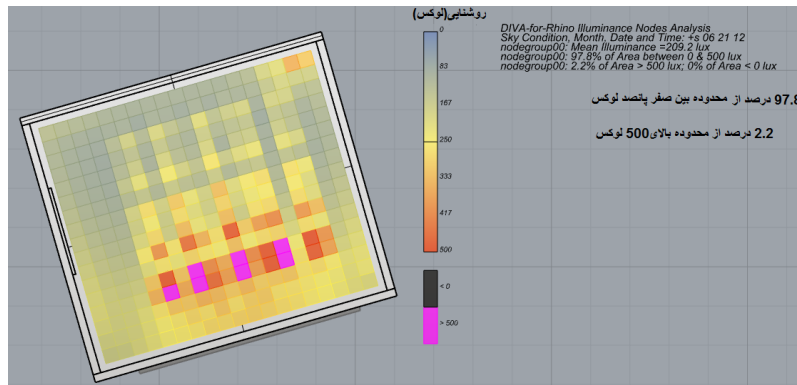
شکل ۱۶- روشنایی کلاس بدون رف نور-حالت پایه، اول تیرماه ساعت ۱۲ ظهر(نگارندگان)
