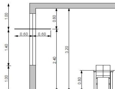
شکل ۷- تیپ یک (رف در وسط)
