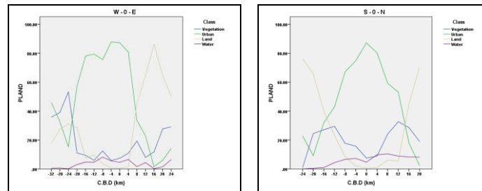
شکل ۶- تغییرات سنجه درصد سیمای سرزمین در سطح کلاس - سال ۲۰۱۸
