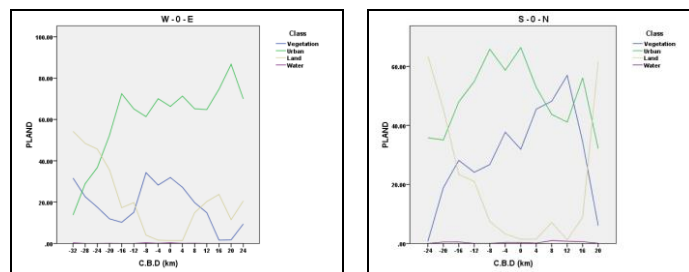
شکل ۵- تغییرات سنجه درصد سیمای سرزمین در سطح کلاس - سال ۲۰۰۸
