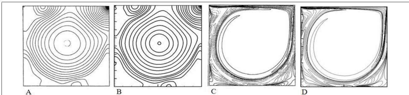
شکل ۱۷. منحنی های هم فشار و هم چرخش برای Re=5000 (A,C) [34] Bruneau and Saad (B,D) روش MCB مرتبه دوم.
