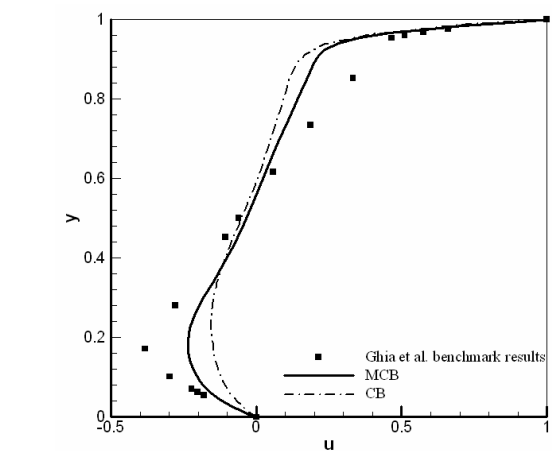
شکل ۴. مقایسه نتایج به دست آمده برای مولفه سرعت u در روی خط عمودی گذرا از مرکز حفره با استفاده از طرح های MCB و CB با دقت مرتبه اول در Re=1000 و شبکه 40 \times 40 .
