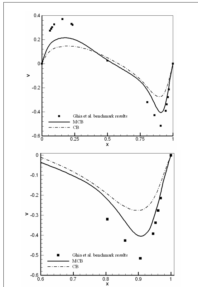
شکل ۵. مقایسه نتایج به دست آمده برای مولفه سرعت v در روی خط افقی گذرا از مرکز حفره با استفاده از طرح های MCB و CB با دقت مرتبه اول در Re=1000 و شبکه 40 \times 40 .
