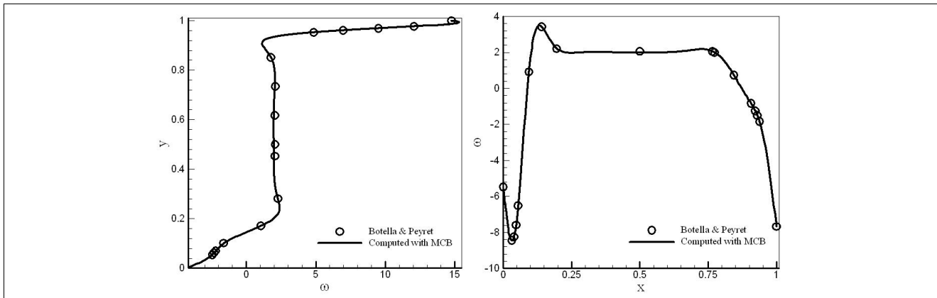
شکل ۲۰. نتایج به دست آمده برای چرخش در روی خطوط افقی و عمودی گذرا از مرکز هندسی حفره در Re=1000 با استفاده از طرح مرتبه دوم در مقایسه با Botella & Peyret [35].
