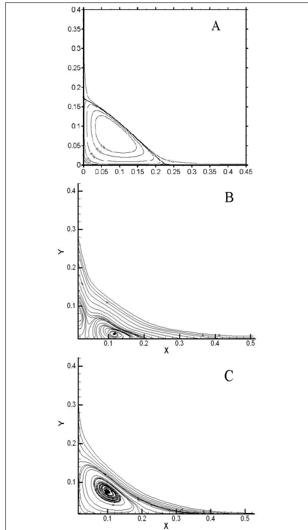
شکل ۱۰. خطوط جریان گردابه گوشه پایین سمت چپ حفره
