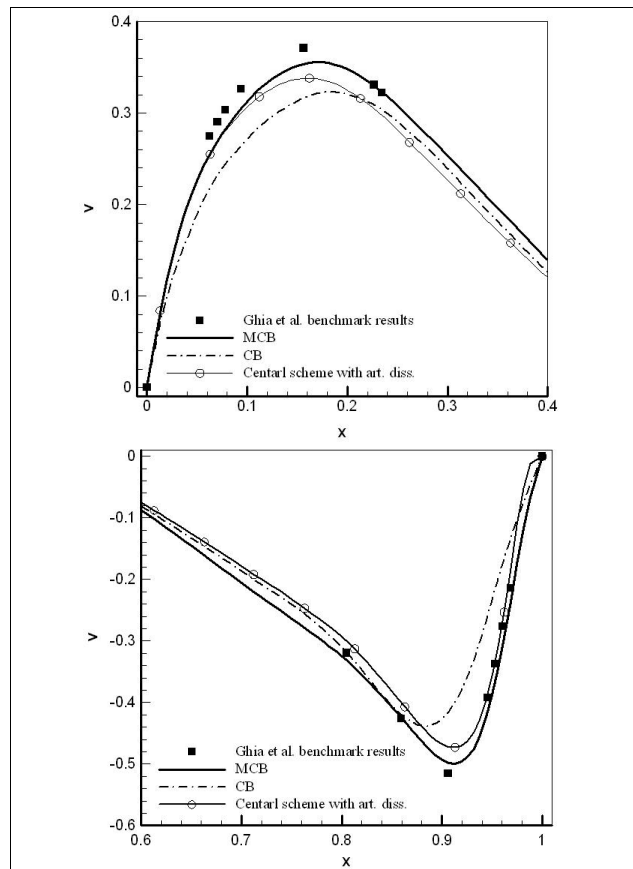
شکل ۸. نمای بزرگ شده بیشینه و کمینه نمودار مولفه سرعت v در روی خط افقی گذرا از مرکز حفره با استفاده از طرح‌های CB و MCB با دقت مرتبه دوم و طرح میانگین گیری مرکزی در Re=1000 و شبکه 40 \times 40 .
