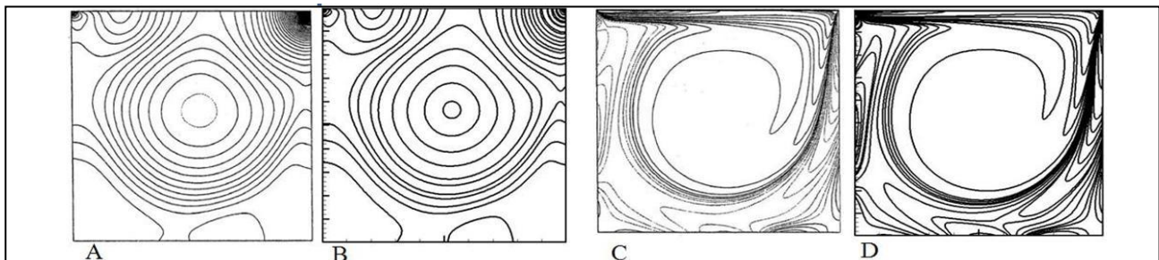
شکل ۱۶. منحنی های هم فشار و هم چرخش برای Re=1000 (A,C) [34] Bruneau and Saad (B,D) روش MCB مرتبه دوم.
