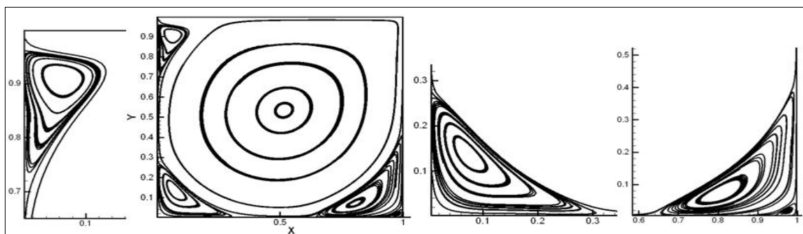
شکل ۱۳. خطوط جریان گردابه های اولیه و ثانویه و نمای بزرگ شده گردابه ها در Re=5000 .
