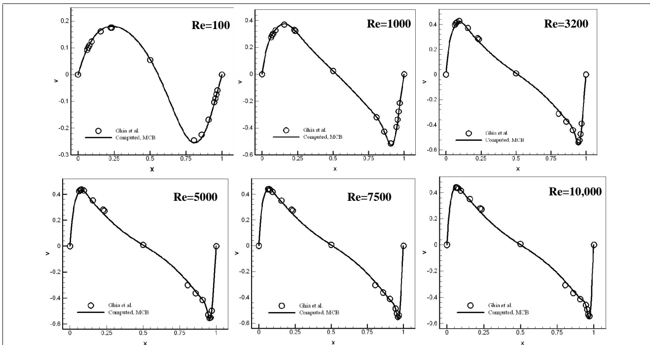
شکل ۱۹. مقایسه مقادیر محاسبه شده برای مولفه سرعت v در روی خط افقی گذرا از مرکز حفره با نتایج مرجع Ghia et al. [27] در اعداد رینولدز مختلف.
