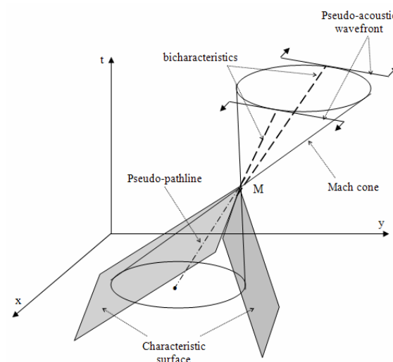
شکل ۱. ساختار مشخصه های معادلات جریان تراکم ناپذیر تصحیح شده با تراکم پذیری مصنوعی.
