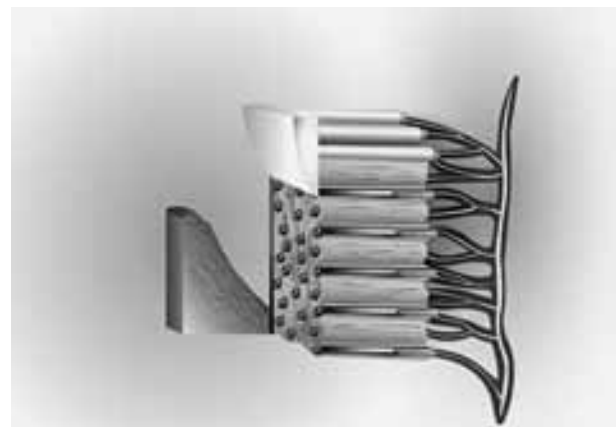
شکل ۱: تئوری هیدرودینامیک
