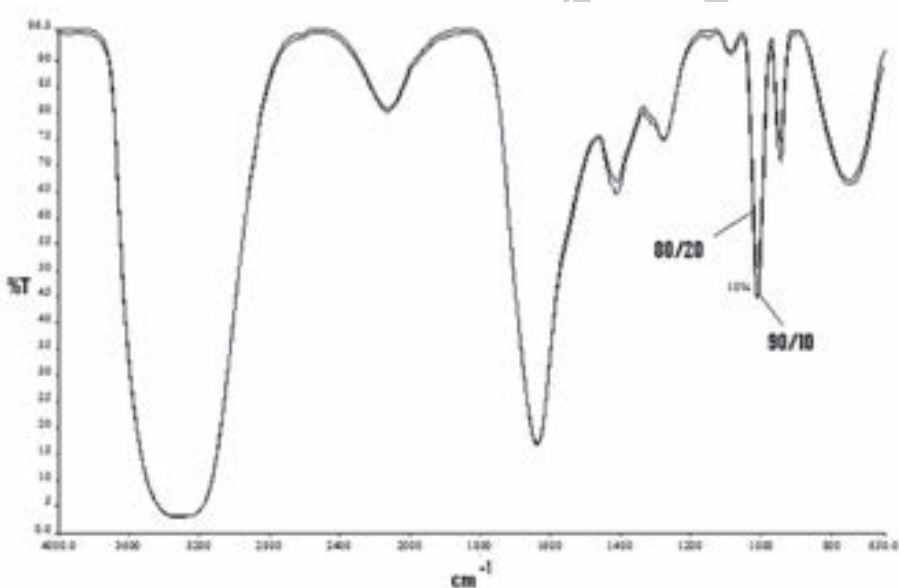
نمودار ۳- نمودارهای FTIR از کامپوزیت CS/PEO با نسبت‌های ۸۰/۲۰، ۹۰/۱۰
