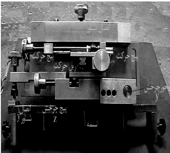
شکل ۲- نمای خلفی از وسیله تثبیت سر
