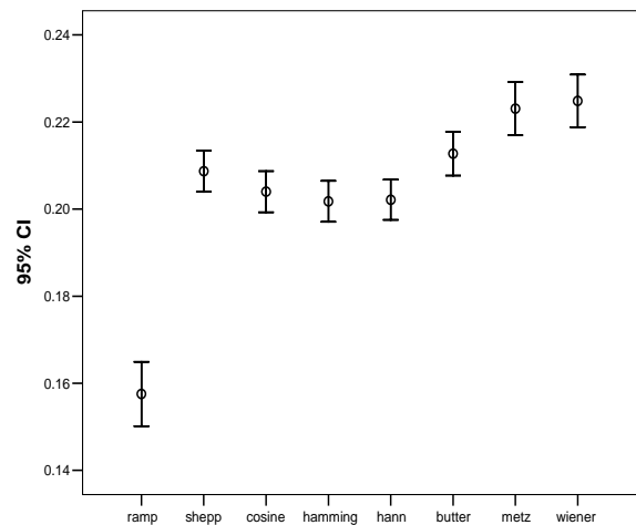
شکل ۴- مقایسه بین فیلترهای Hanning , Hamming , Shep-Log , Cosine بدون توجه به نوع کلیماتور و میزان شمارش است و میانگین شاخص کلی کیفیت تصویر به همراه فاصله اطمینان را برای کلیه فیلترها در فانتوم سه بعدی (چهار مقطع) نمایش می دهد.
