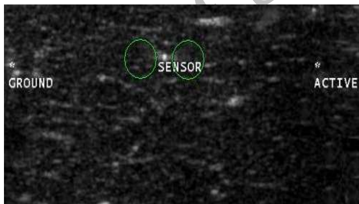
شکل ۳- محل قرار گیری الکترودها و حسگر حرارتی در یک تصویر فوآصوت
